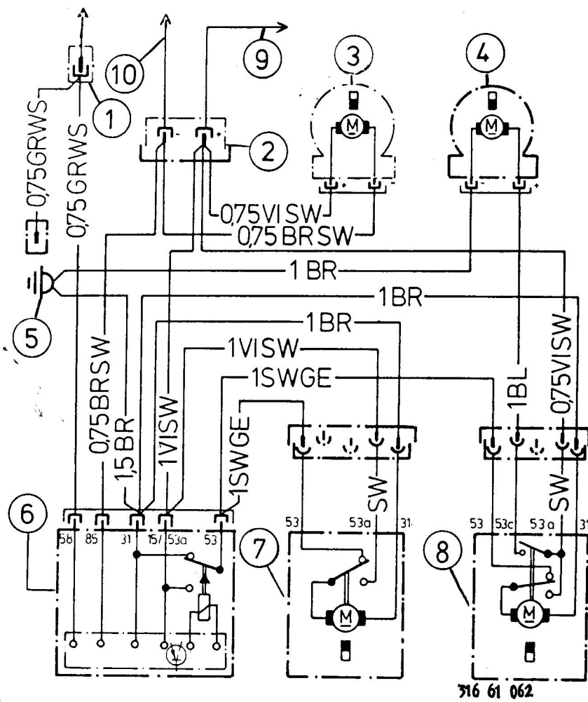
Schaltplan für Scheinwerfer-Reinigungsanlage BMW 316 – 320 i
